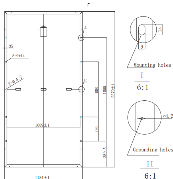
Рисунок 1 – схематическое изображение ФЭМ
