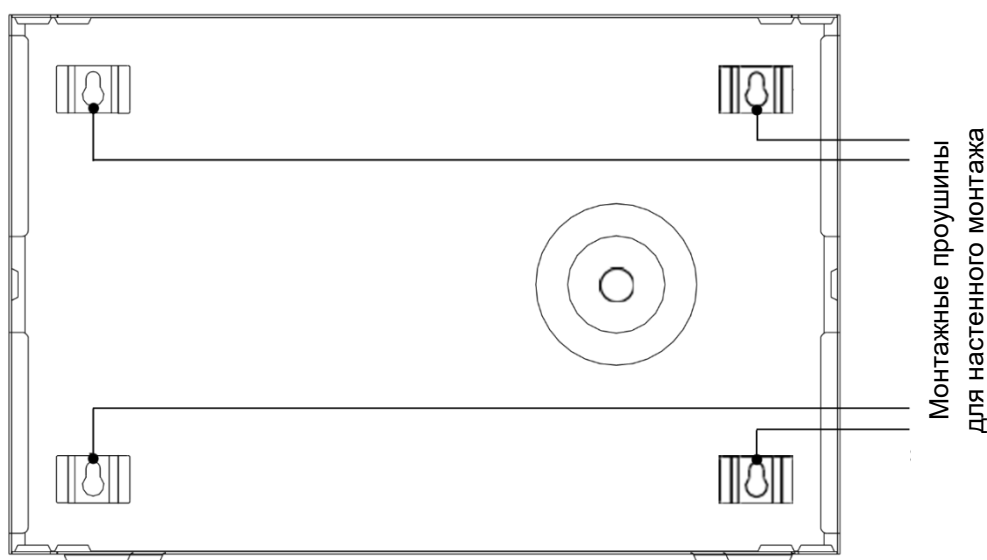
Рисунок 5. Крепления для настенного монтажа стабилизатора.
