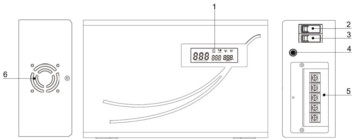
Рисунок 3. Внешний вид стабилизаторов напряжения SMARTWATT AVR SLIM 3000-5000VA. Описание элементов приводится в таблице 3.
